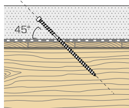
Montáž pri 45° so zvukotesnou membránou.
