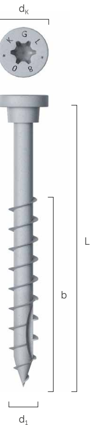
KGL EVO Ø8
